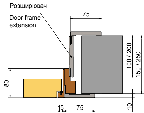
Алюмінієвий короб iDoors "INSIDE" зворотного відкриття
