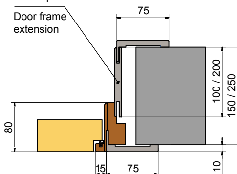
Алюмінієвий короб iDoors "INSIDE" зворотного відкриття Aluminum door frame iDoors "INSIDE" reverse opening
