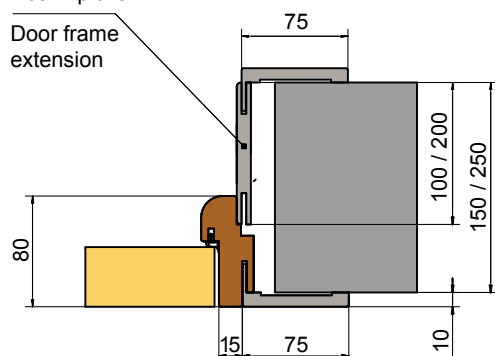
Алюмінієвий короб iDoors "Стандарт" зовнішнього відкриття Aluminum door frame iDoors "Standard" external opening
