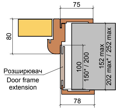
Алюмінієвий короб iDoors "INSIDE" зворотного відкриття
