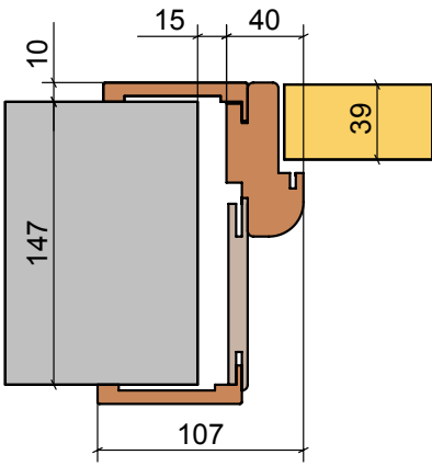
Алюмінієвий короб iDoors "Стандарт" зовнішнього відкриття
