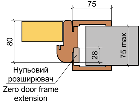
Короб "Компланарний" Door frame "Coplanar"
